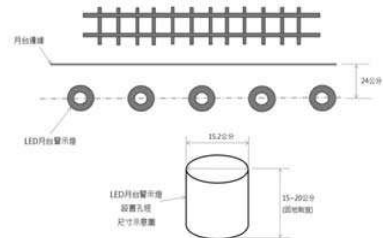
圖3.10.4 LED月台警示燈位置示意圖
