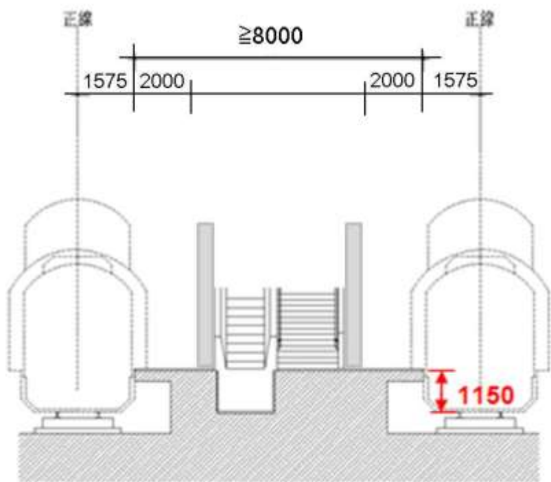
月台上構造物距月台邊緣寬度 (單位：mm)
